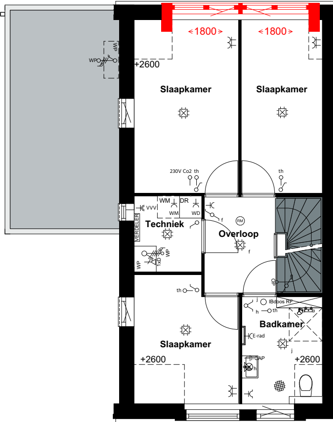
21 - 23 EERSTE VERDIEPING
