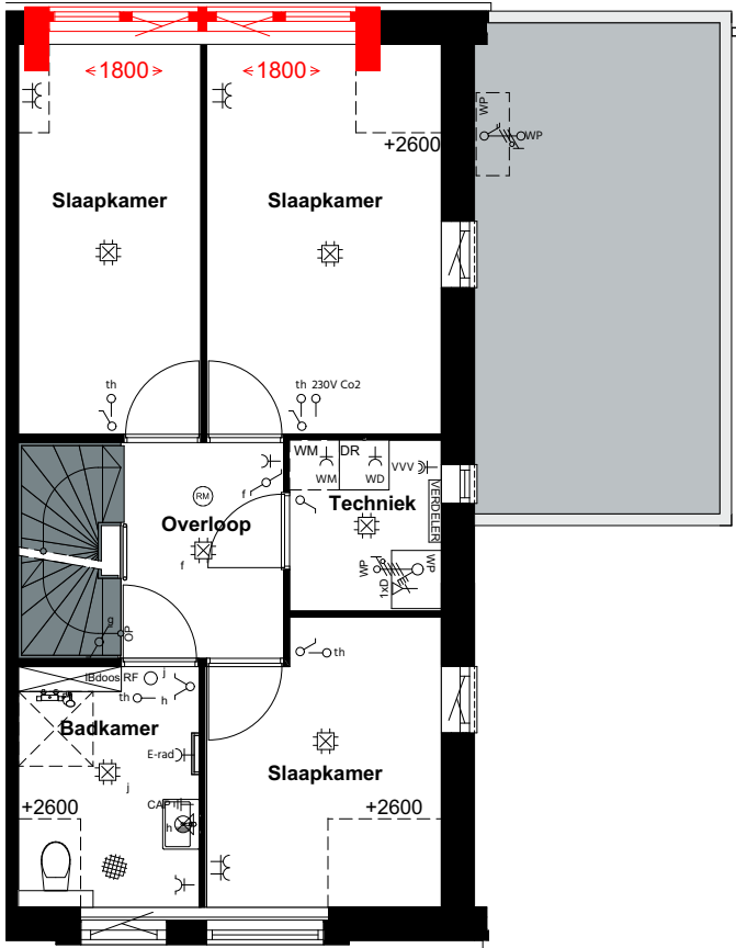
22 - 24 EERSTE VERDIEPING
